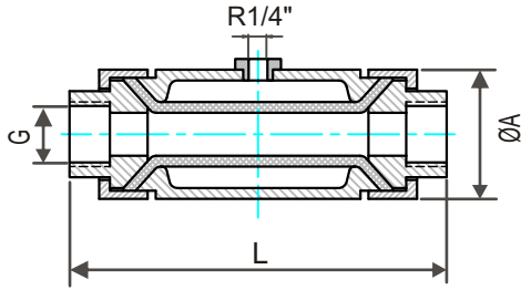
Dişli Pinch Valf
